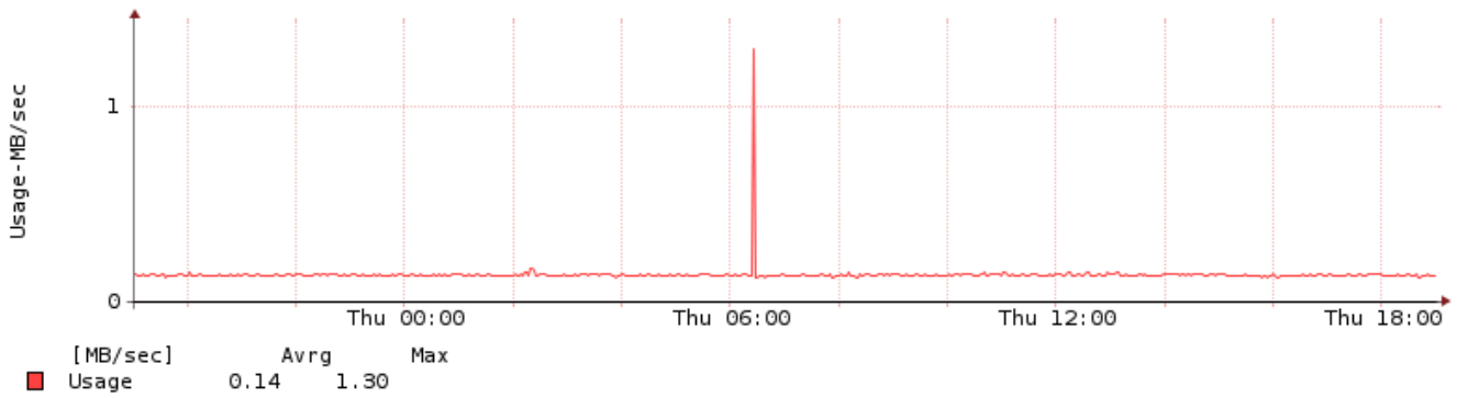
Disk : controller : 19:00:00 12.10.2016 - 19:00:00 13.10.2016
