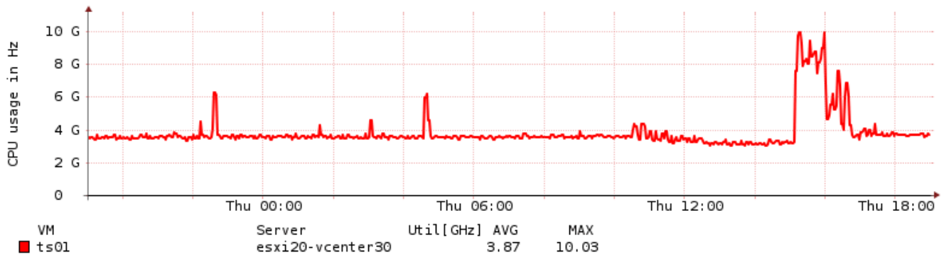
VM: ts01 : 19:00:00 12.10.2016 - 19:00:00 13.10.2016
