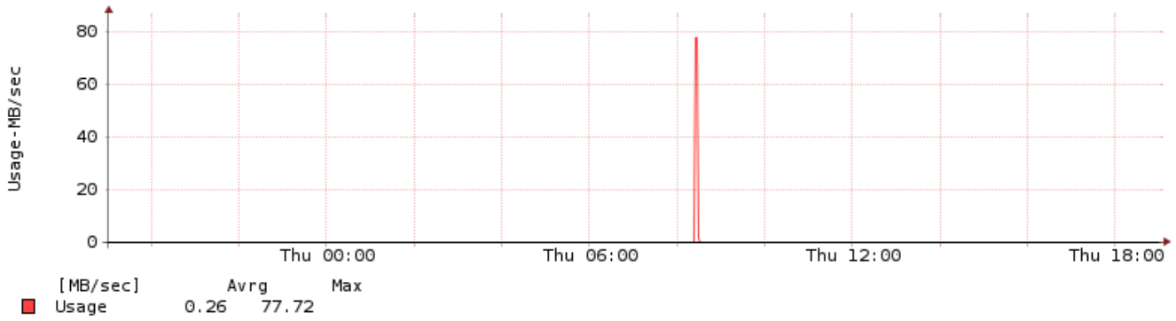
Disk : chef : 19:00:00 12.10.2016 - 19:00:00 13.10.2016
