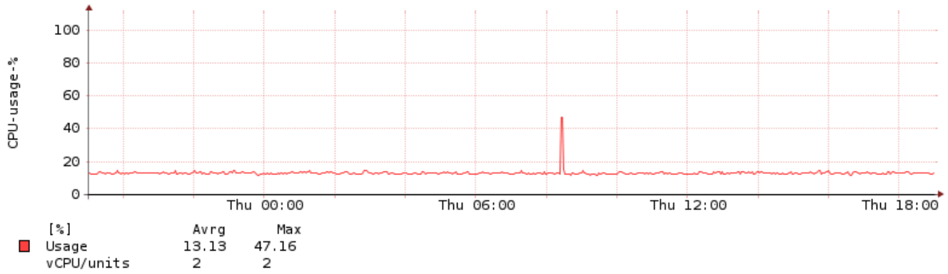
VM : chef : 19:00:00 12.10.2016 - 19:00:00 13.10.2016
