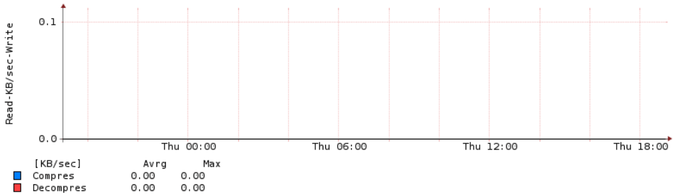
VM : ts01 : 19:00:00 12.10.2016 - 19:00:00 13.10.2016
