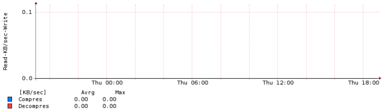
VM : chef : 19:00:00 12.10.2016 - 19:00:00 13.10.2016
