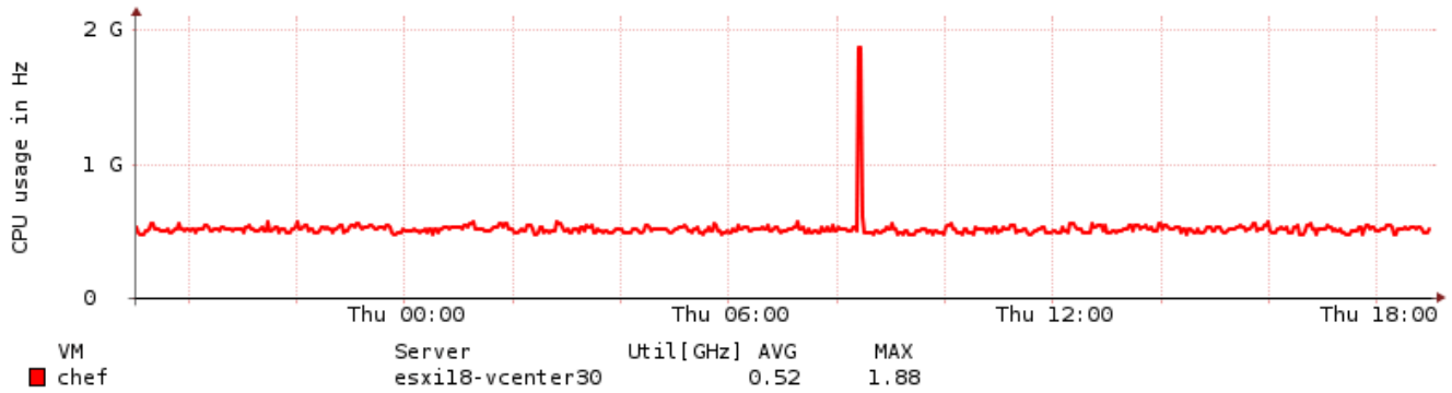
VM: chef : 19:00:00 12.10.2016 - 19:00:00 13.10.2016
