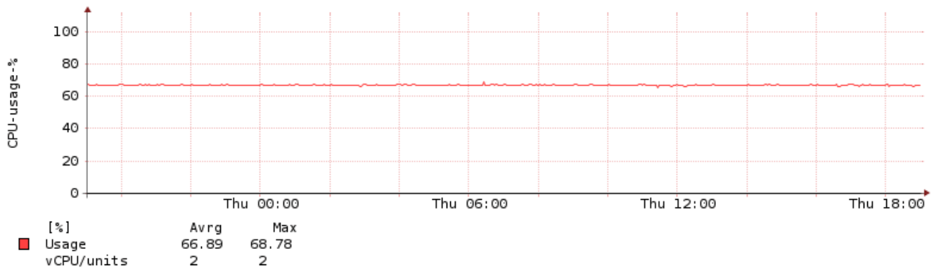
VM : controller : 19:00:00 12.10.2016 - 19:00:00 13.10.2016
