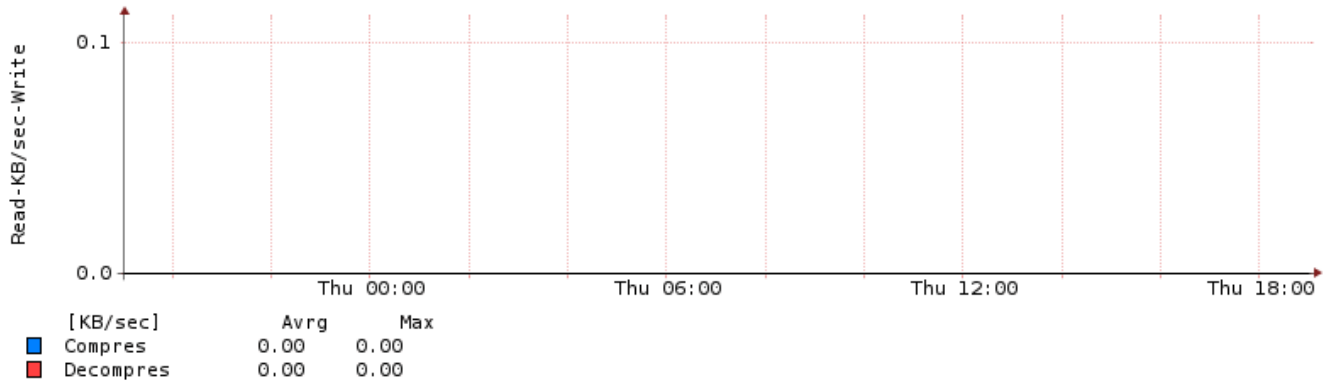
VM : ICN : 19:00:00 12.10.2016 - 19:00:00 13.10.2016
